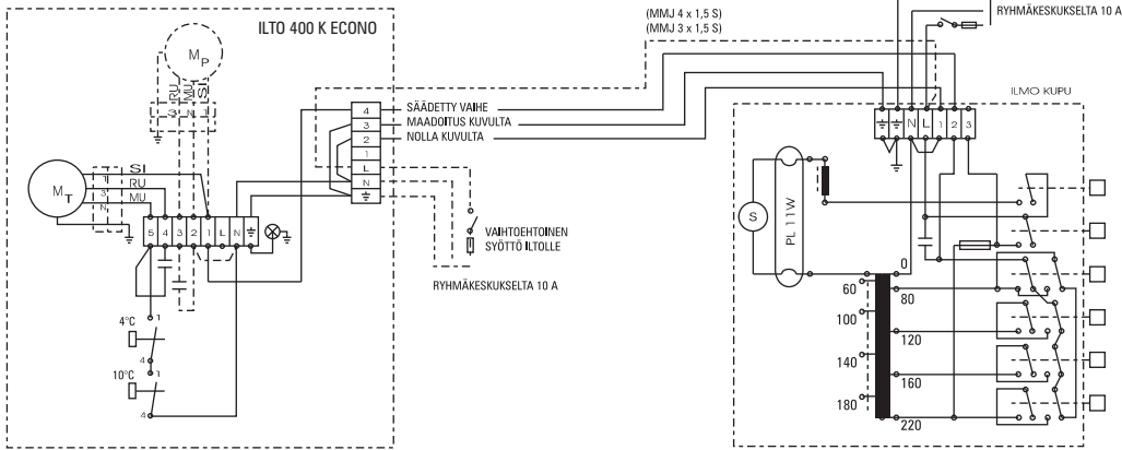
LIESIKUPOHJAUS SYÖTÖ KUVULLE TAI ILTOLLE ILTO 400 K Econo
