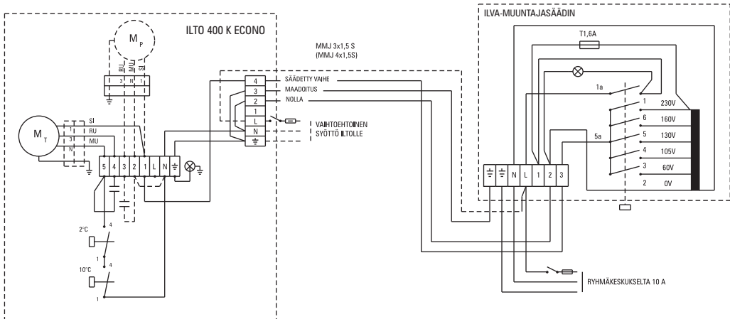
ERILLISSÄÄDINOHJAUS SYÖTÖ SÄÄTIMELLE TAI ILTOLLE ILTO 400 K Econo ILVA-MUUNTAJASÄÄDIN
