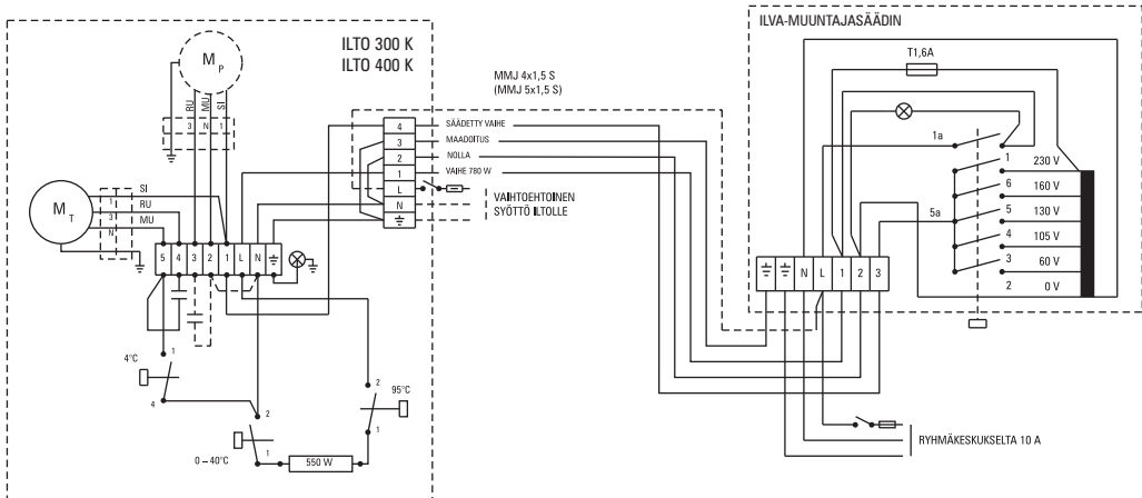
ERILLISSÄÄDINOHJAUS SYÖTÖ SÄÄTIMELLE TAI ILTOLLE ILTO 300 K, ILTO 400 K ILVA-MUUNTAJASÄÄDIN
