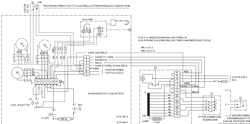
ERILLISSÄÄDINOHJAUS SYÖTÖ SÄÄTIMELLE TAI ILTOLLE ILTO 300 K, ILTO 400 K ILVA K -MUUNTAJASÄÄDIN
