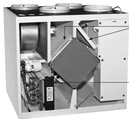
Karkeasuodatin (mahd. teksti tai väri alapuolella)
