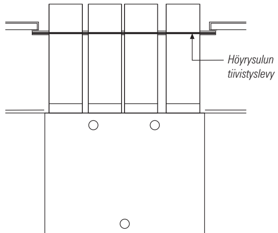
Höyrösulun tiivistyslevyn tiivistemattoon leikataan käyttöön tulevien lähtöjen kohdalle halkaisijaltaan n. 10 mm pienempi aukko.
