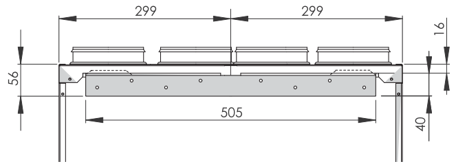
Seinäasennustelineen mitat
