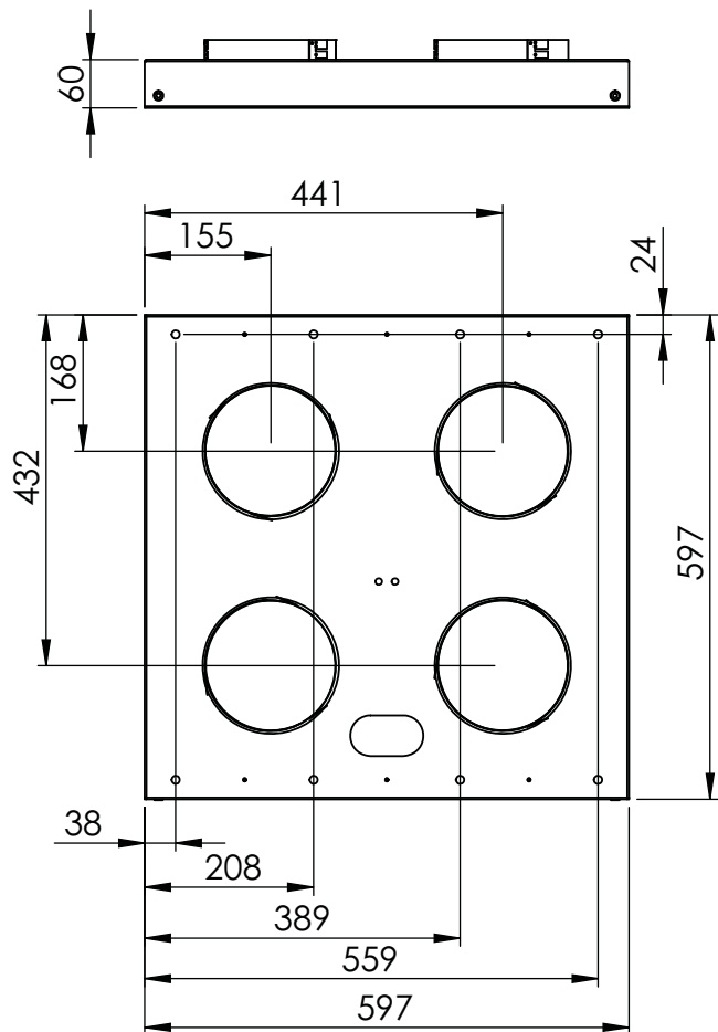
Kattoasennustelineen mitat
