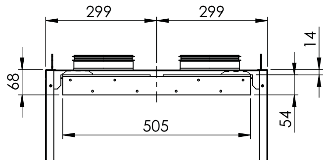
Seinäasennustelineen mitat
